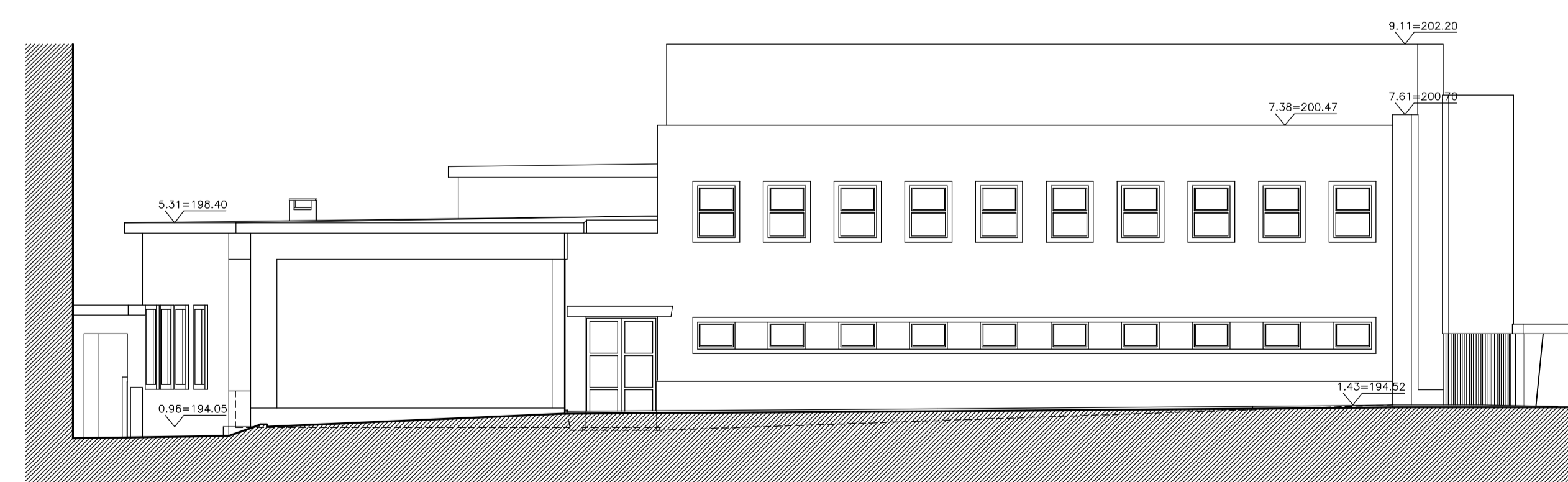
ALÇADO LATERAL ESQUERDO (RUA VASCO DA GAMA)
