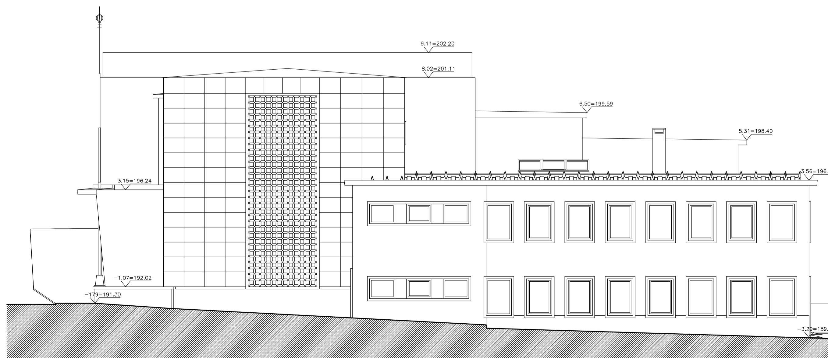
ALÇADO LATERAL DIREITO (RUA INFANTE D. HENRIQUE)
